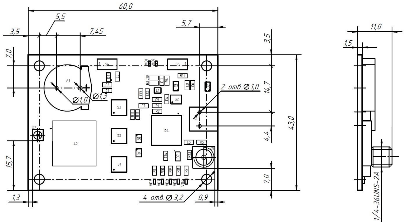
Рисунок 2 – Сборочный чертёж аппаратуры ПРО-04
