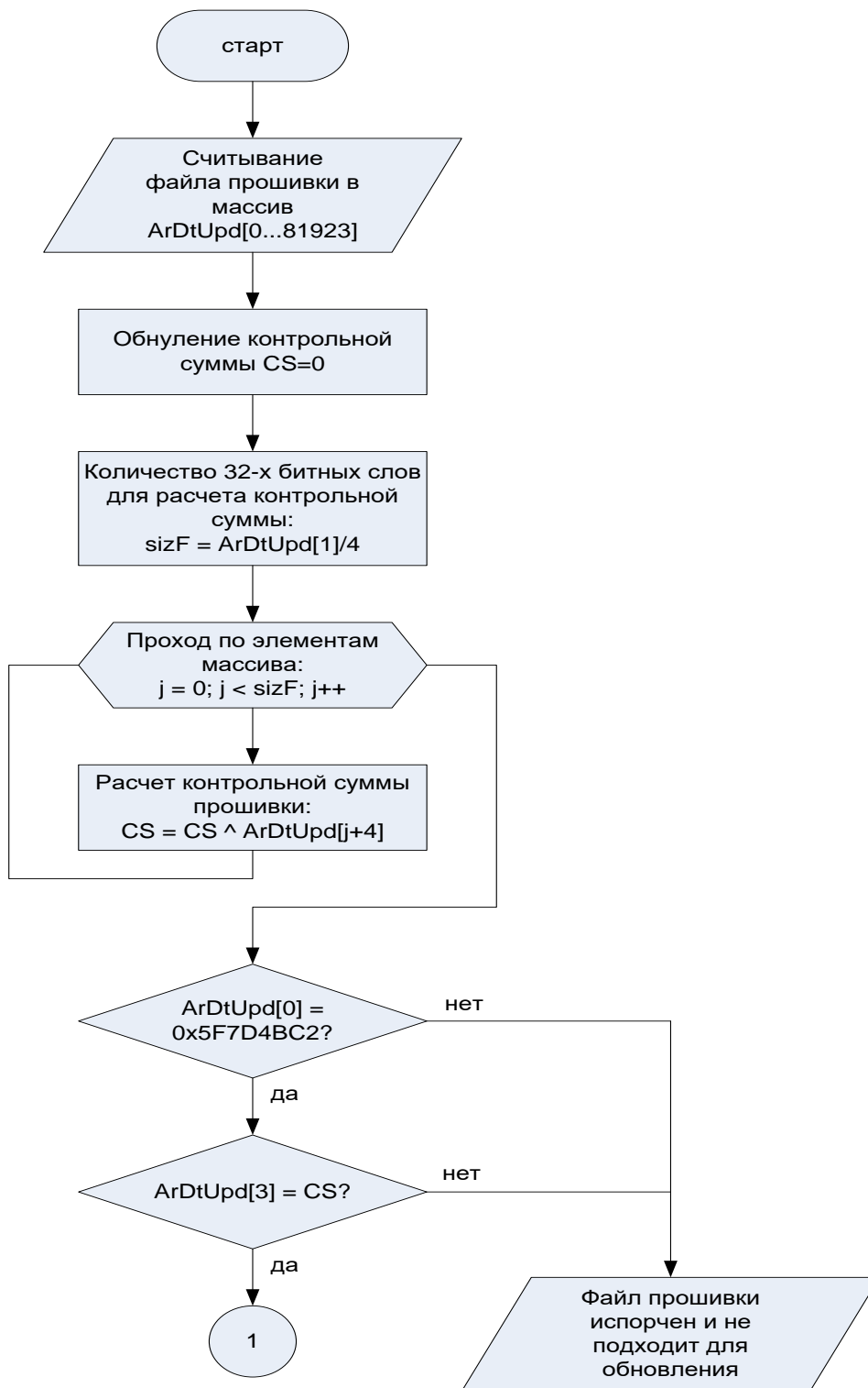
Рисунок 10 – Процедура подготовки массива данных ПО
