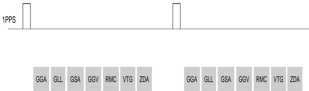
Рисунок 7 – Последовательность выдачи NMEA сообщений
