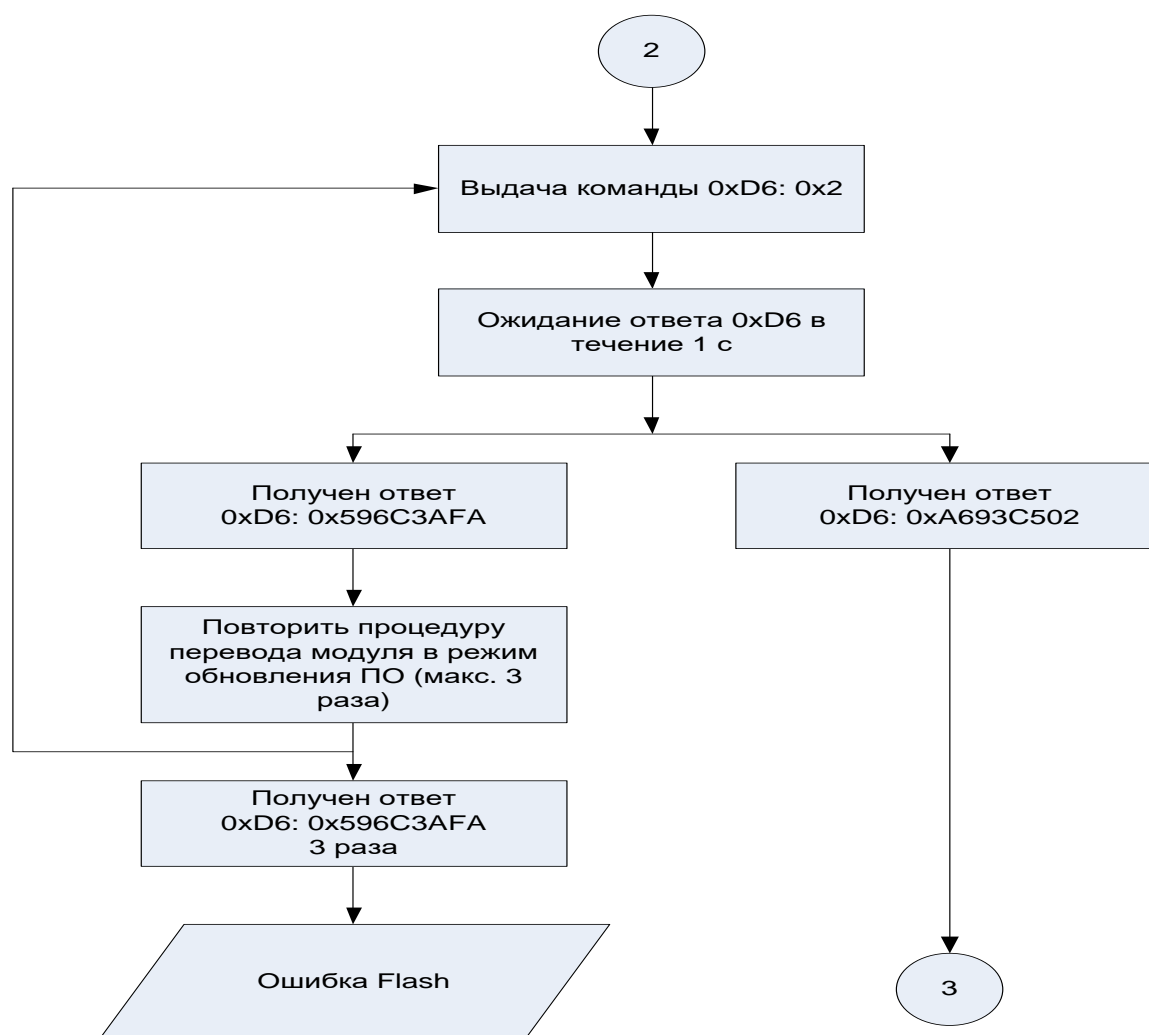
Рисунок 12 – Процедура верификации стирания Flash памяти
