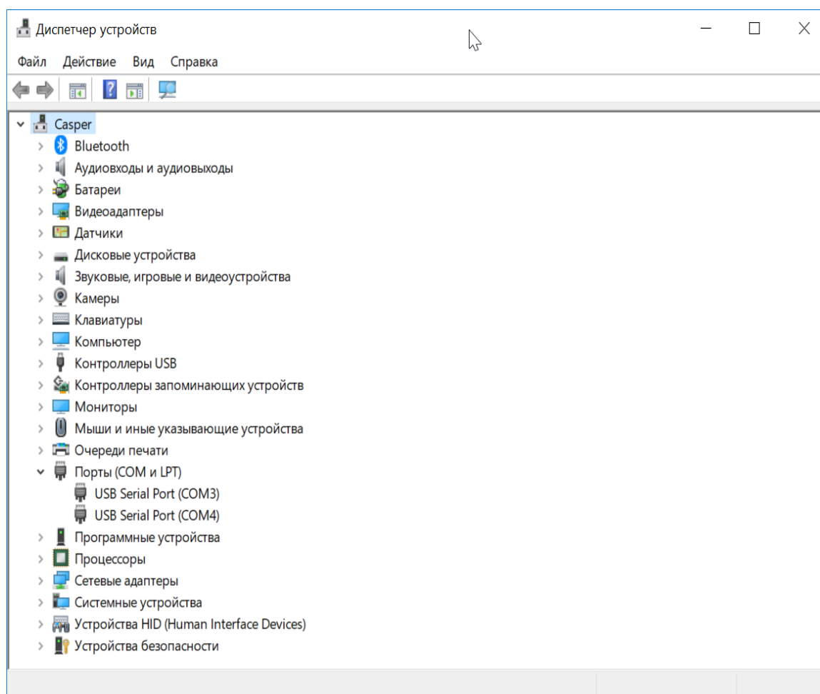
Рисунок 6 – Вид диспетчера устройств после подключения аппаратуры ПРО-04 к ПК
