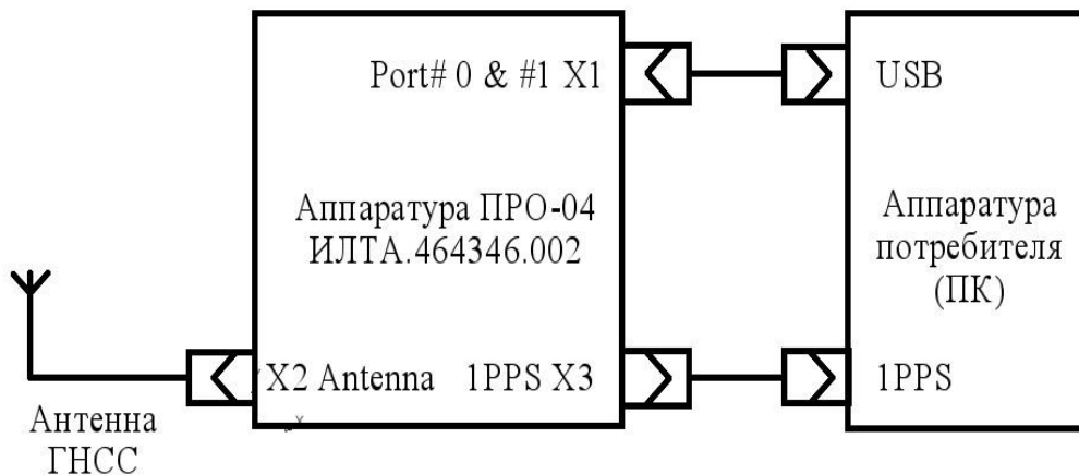
Рисунок 4 – Типовая схема подключения аппаратуры ПРО-04
