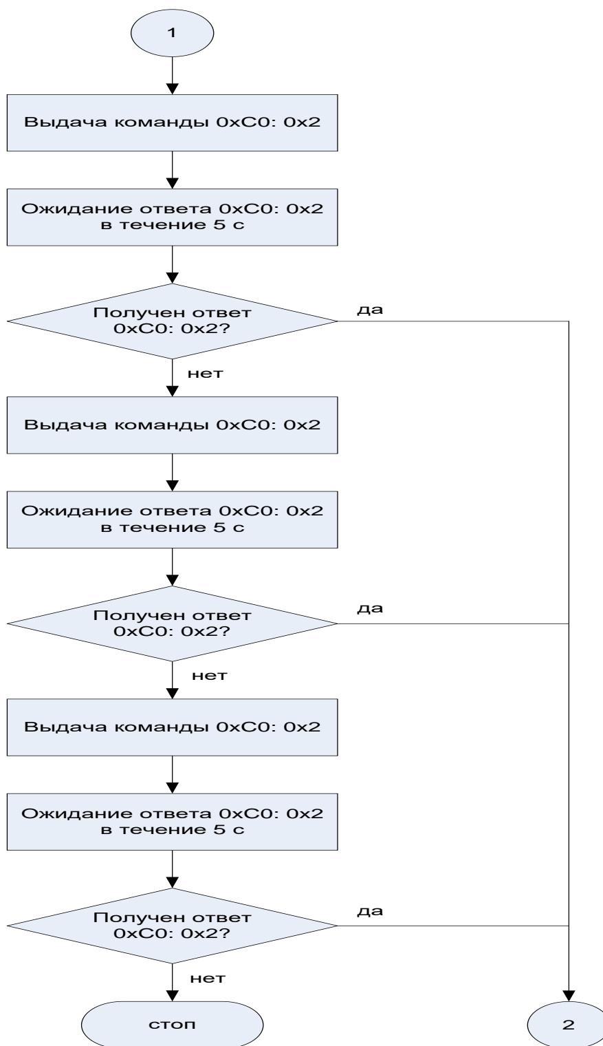
Рисунок 11 – Процедура перевода аппаратуры ПРО-04 в режим обновления ПО
