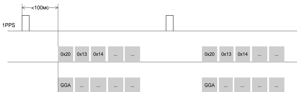
Рисунок 8 – Временная привязка сообщений к секундной метке времени
