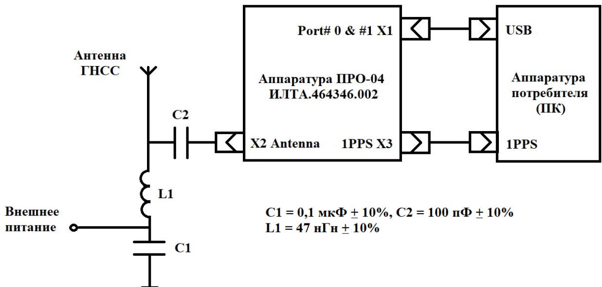
Рисунок 5 – Типовая схема подключения аппаратуры ПРО-04 с внешним питанием антенны
