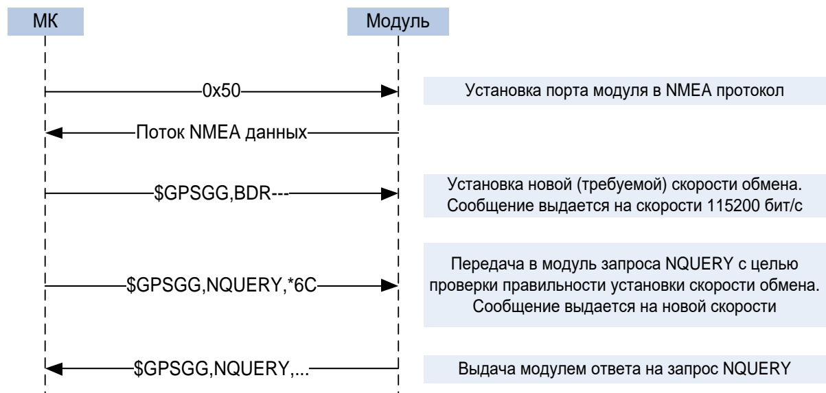
Рисунок 15 – Последовательность переключения из бинарного протокола в NMEA
