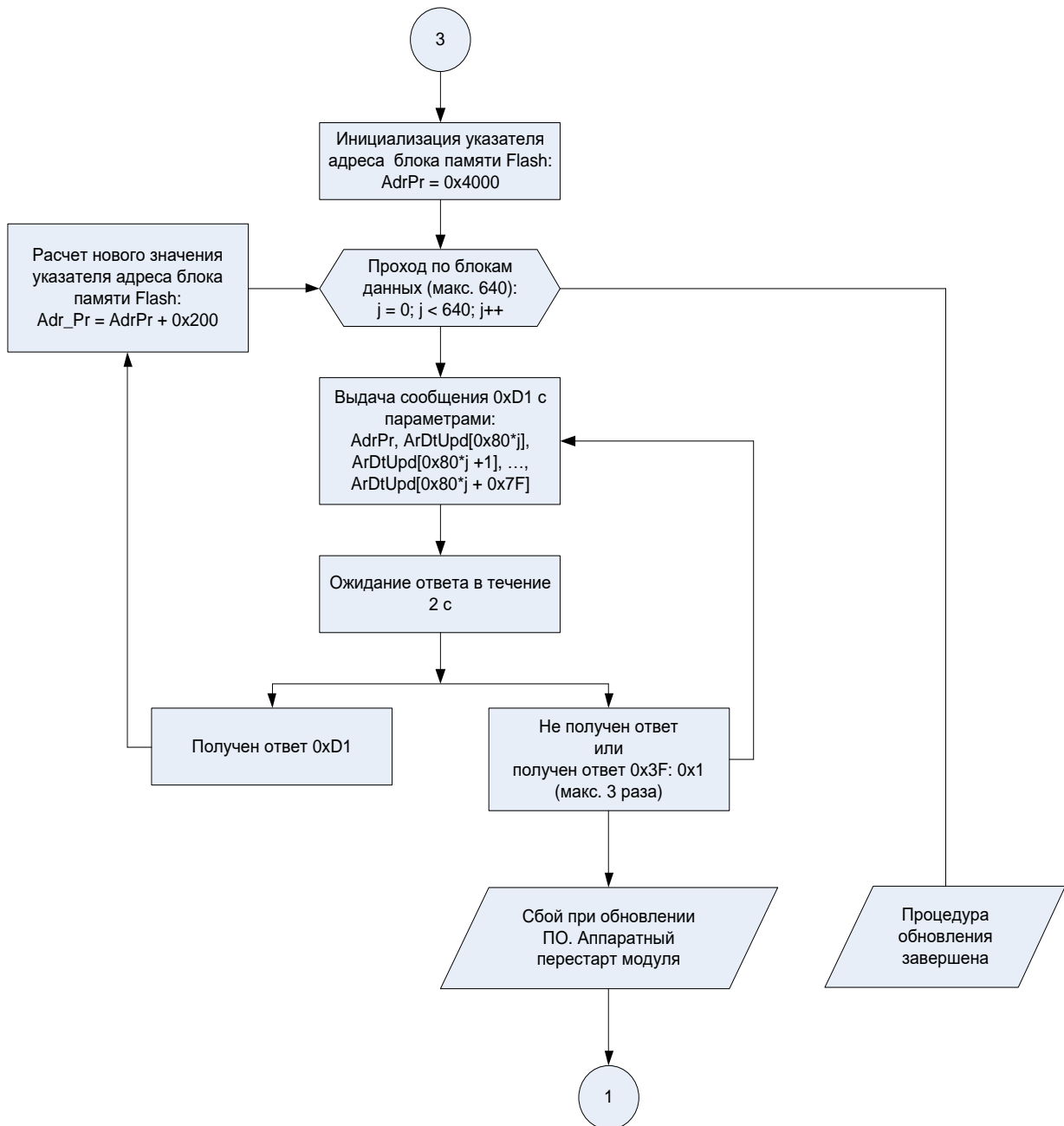
Рисунок 13 – Процедура передачи в аппаратуру ПРО-04 блоков данных
