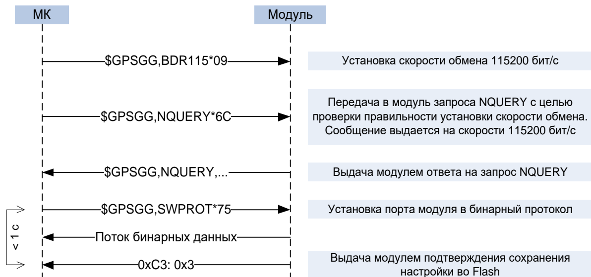
Рисунок 14 – Последовательность переключения из NMEA протокола в бинарный
